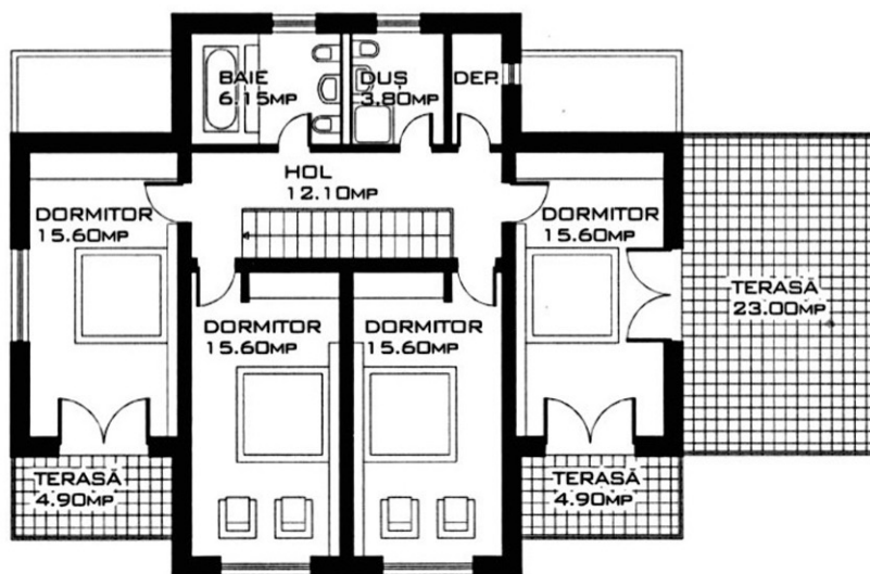
PLAN ETAJ
