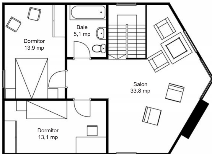
PLAN ETAJ
